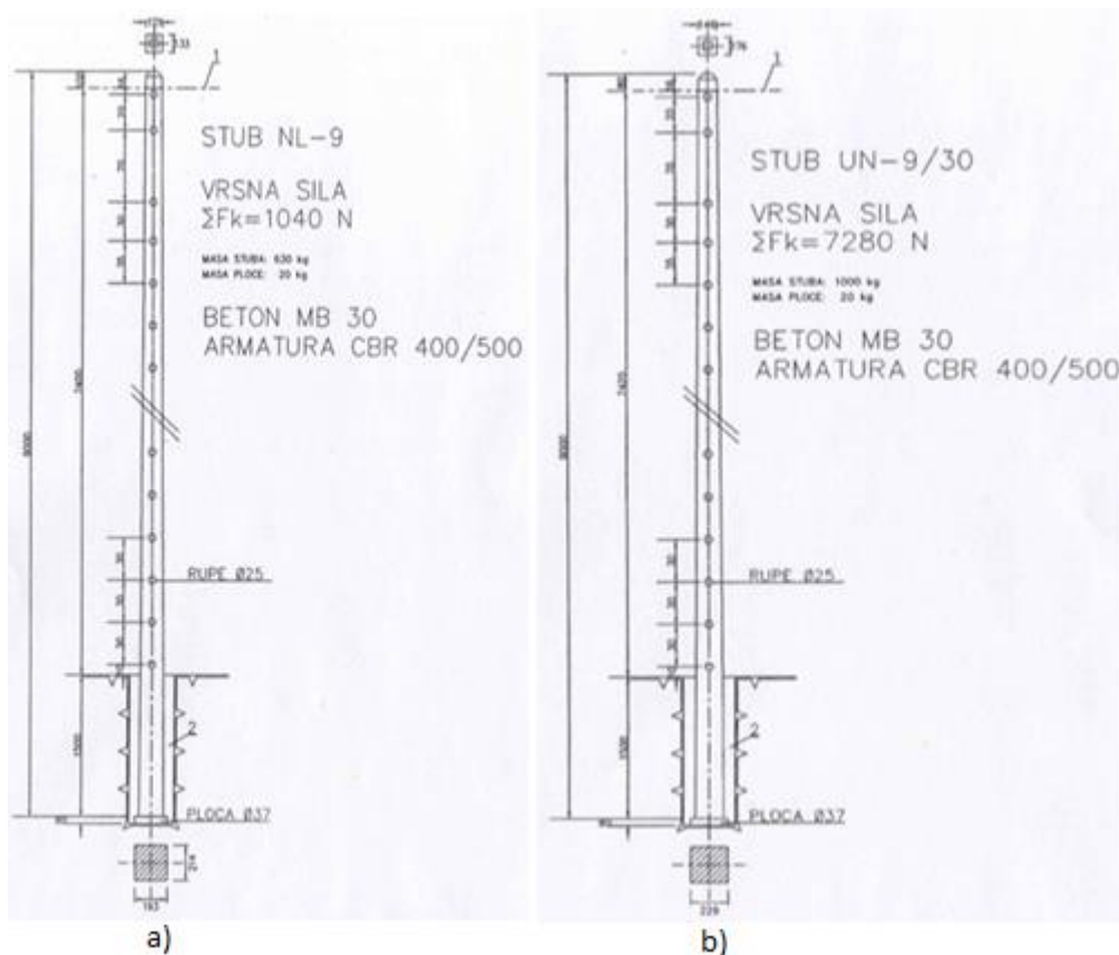
SLIKA 2 - IZGLLED STUBOVA SA VRŠNIM SILAMA A) STUB NL 9 I B) STUB UN-9/30
